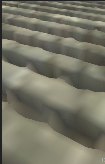
Steps : 32
